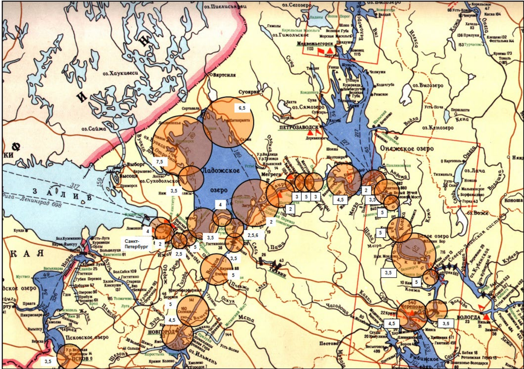
Радиосеть диспетчерского регулирования движения на 2024 г.
