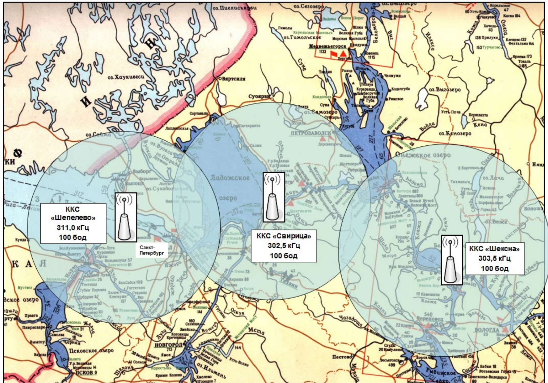
Зоны приема сигнала дифференциальных поправок ГЛОНАСС/GPS на 2024 г.
