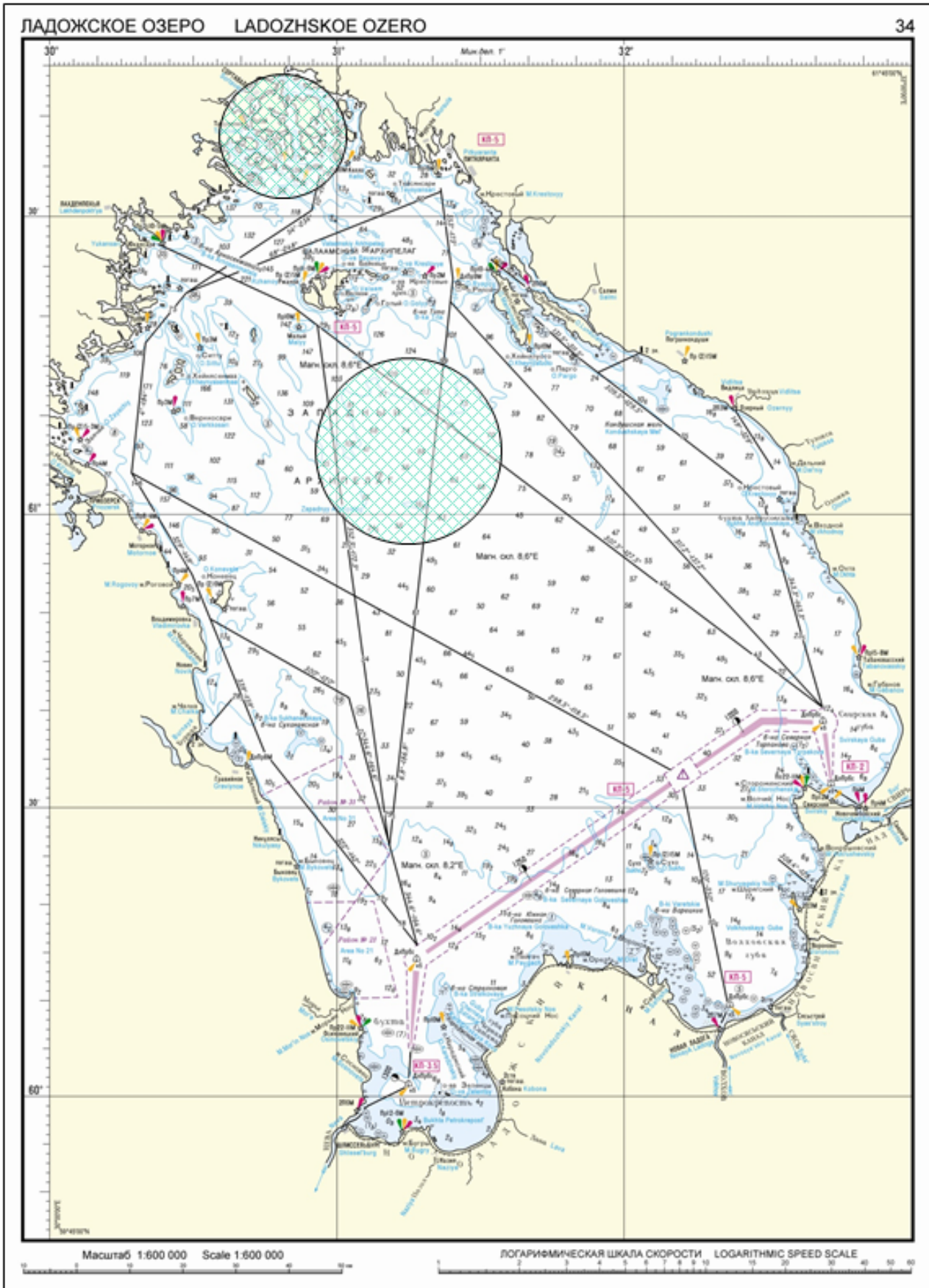
Мертвые зоны» УКВ-радиосвязи на Ладожском озере (2024 г.)
