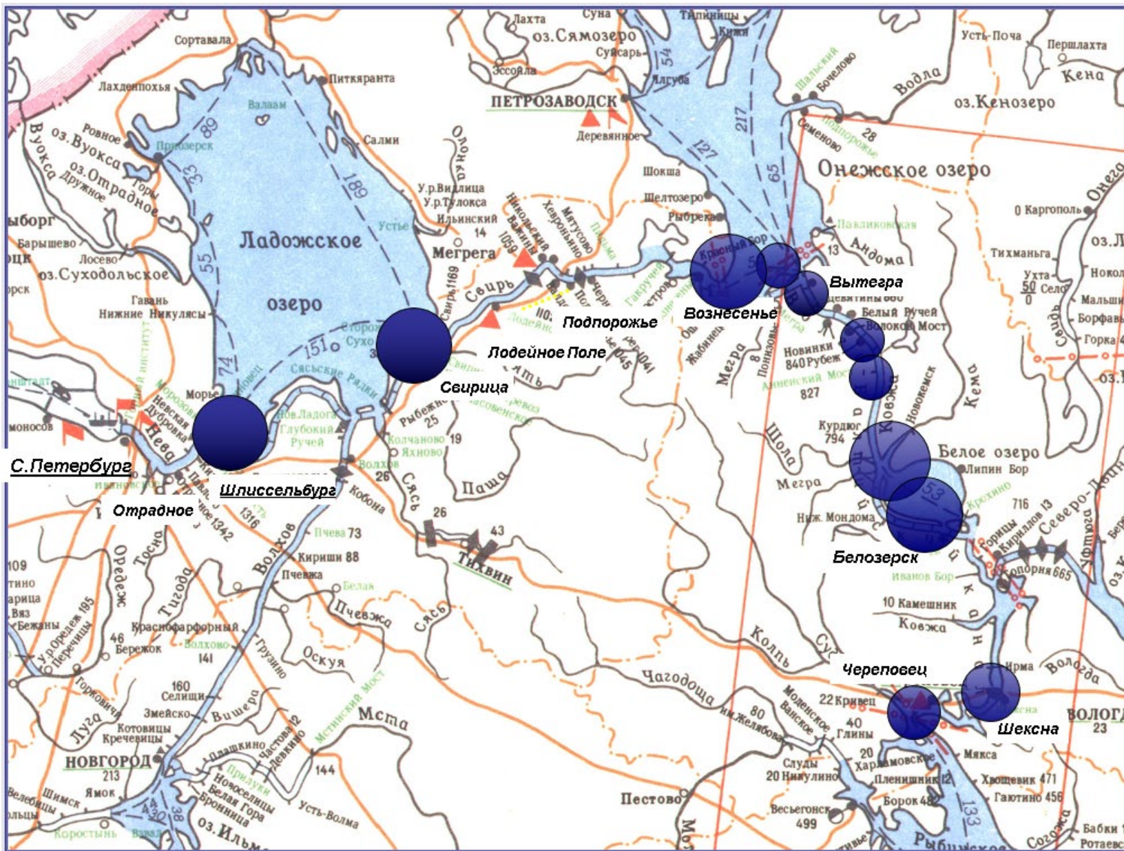
Зоны покрытия береговых радиолокационных станций на 2024 г.
