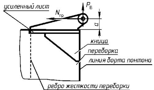
Рис. П3.3.2.4. Схема подкрепления под палубный шарнир и приложения нагрузок
