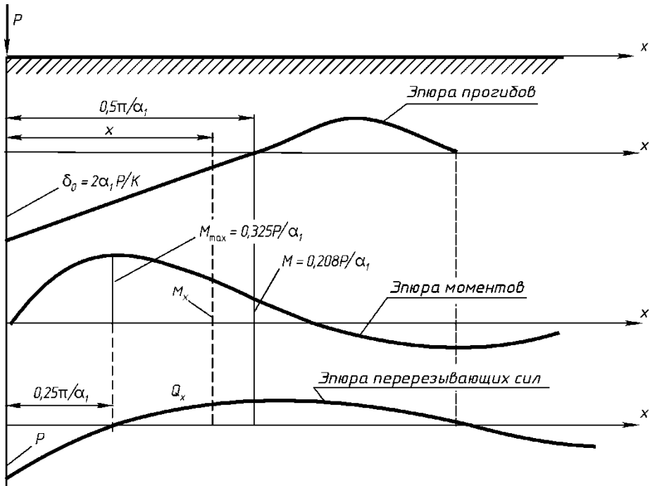
Рис. ПЗ.1.2.1. Эпюры усилий и прогибов в оконечности моста
