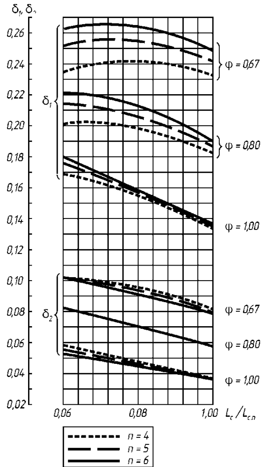
Рис. 4.3.44-3. Коэффициенты \delta_1, \delta_2 при n = 4; 5; 6
