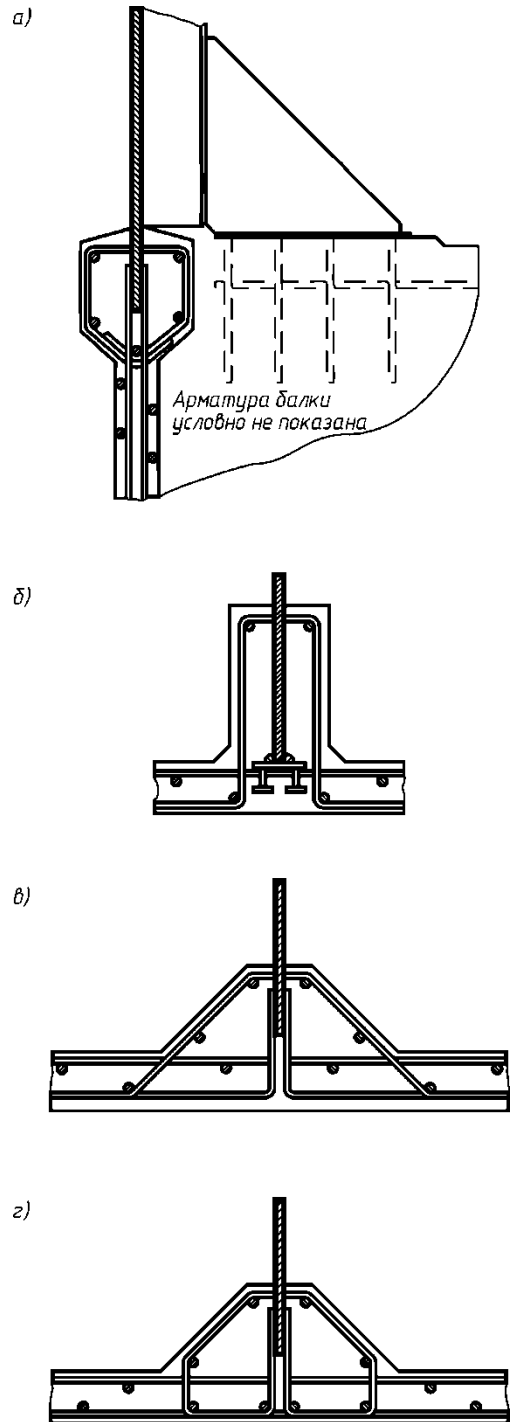
Рис. 4.3.12. Приваривание стенок и переборок к сплошным закладным деталям
