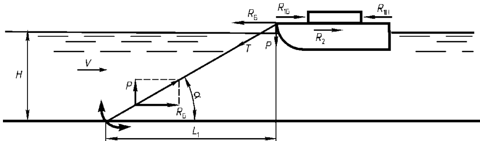
Рис. 8.2.7. Схема якорного раскрепления
