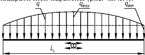
Рис. 4.3.43.4. Эпюра распределения доковой массы:
